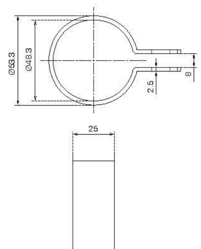
N292 不锈钢支架 N292 SS Side Brackets
